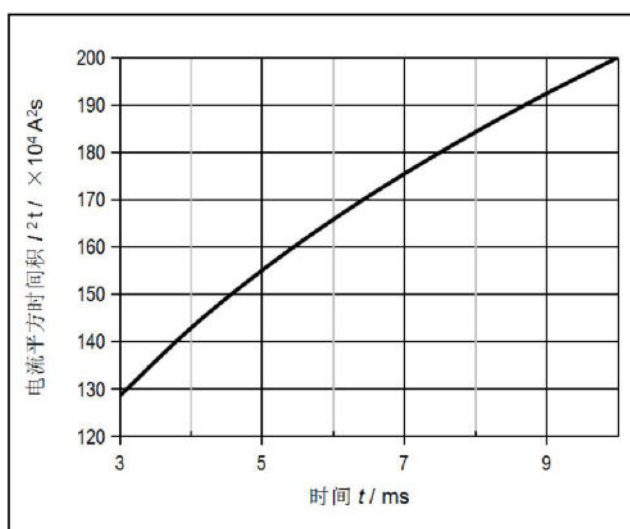
图4. I^2t 特性曲线
