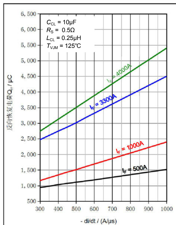
图6. 反向恢复电荷与 -di/dt 的关系曲线
