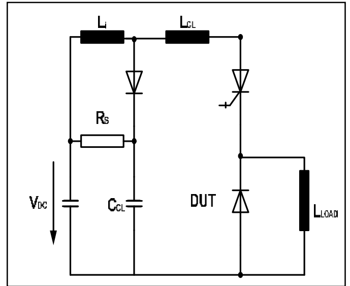
图9. 测试电路示意图
