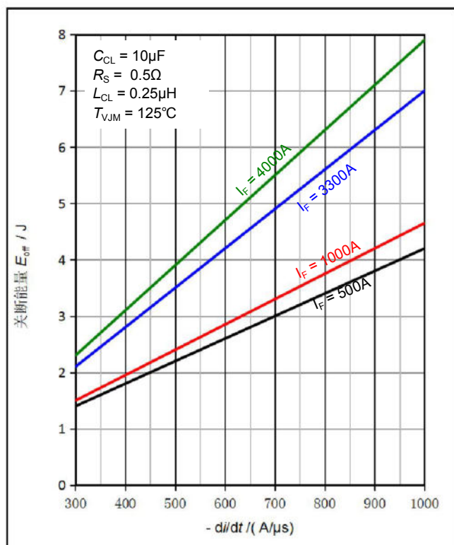
图5. 关断能量与 -di/dt 的关系曲线
