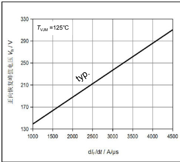
图8. 正向恢复峰值电压与 dI_F/dt 的关系曲线
