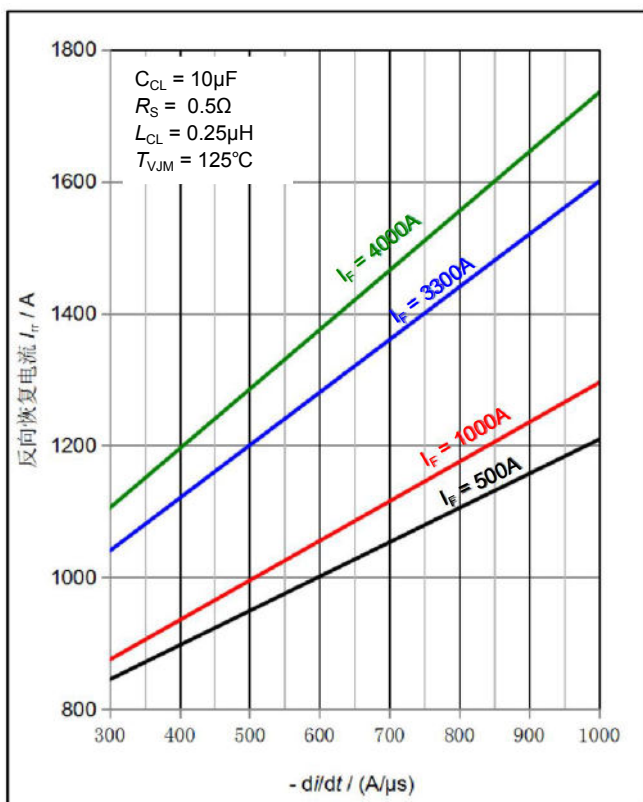
图7. 反向恢复电流与 -di/dt 的关系曲线
