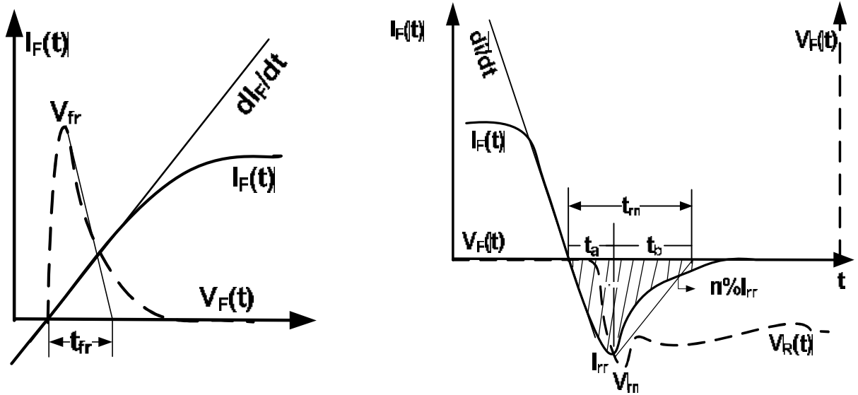
图10. 常规电流电压波形
