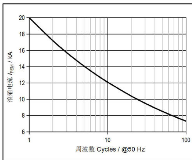
图3. 浪涌电流与周波数的关系曲线
